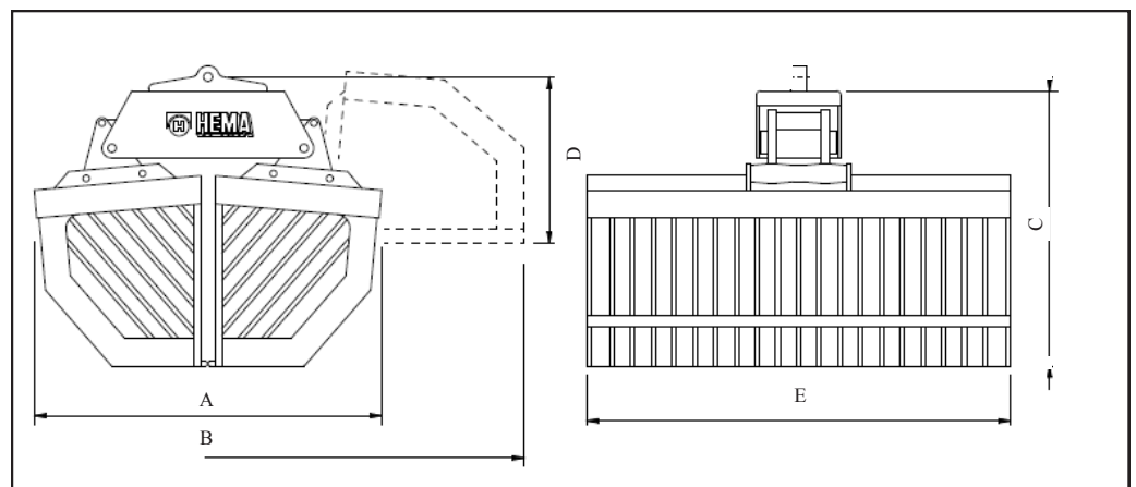
HEMA Sugarbeet Basket RK90-2500
